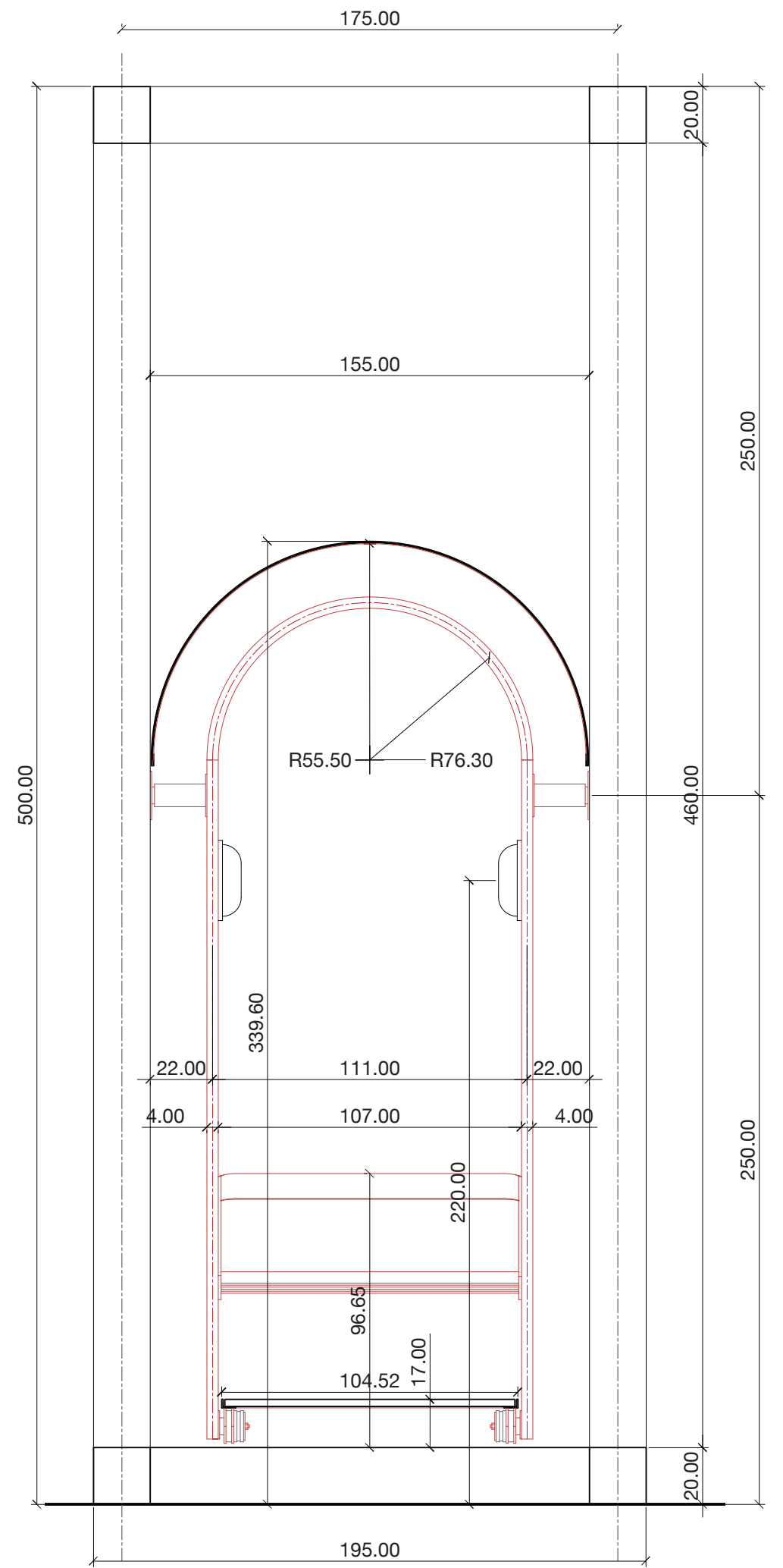
SECTION 2 1:20
